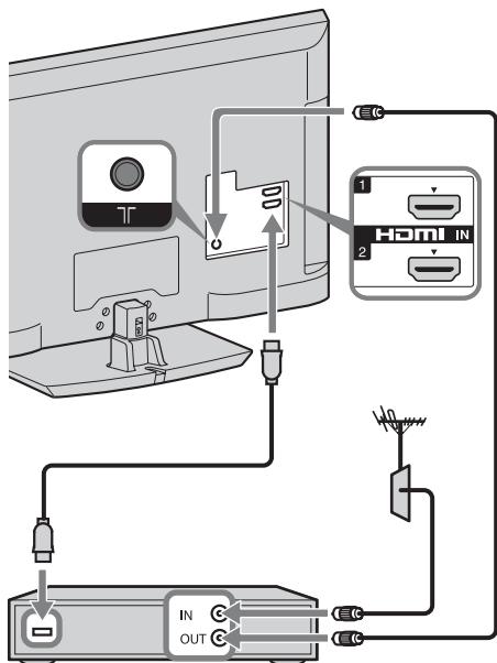
Set Top Box/rekordér (napr. rekordér DVD)
