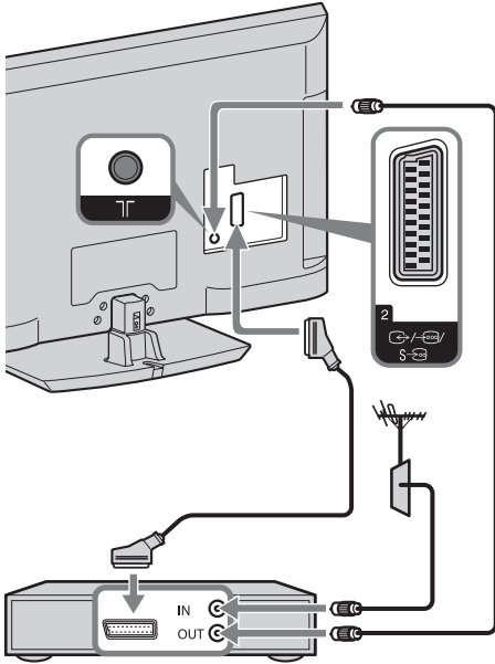
Set Top Box/συσσκευής εγγραφής (π.χ. συσκευή εγγραφής DVD)
