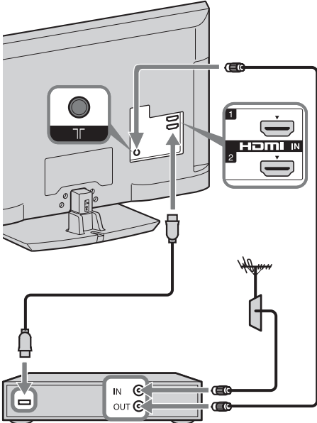
Dijital uydu alıcısı/kaydedici (örn. DVD kaydedici)
