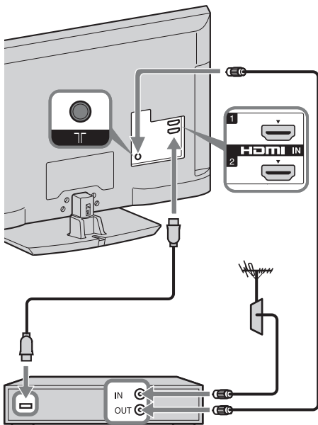
Set Top Box, felvevő (pl. DVD-felvevő)
